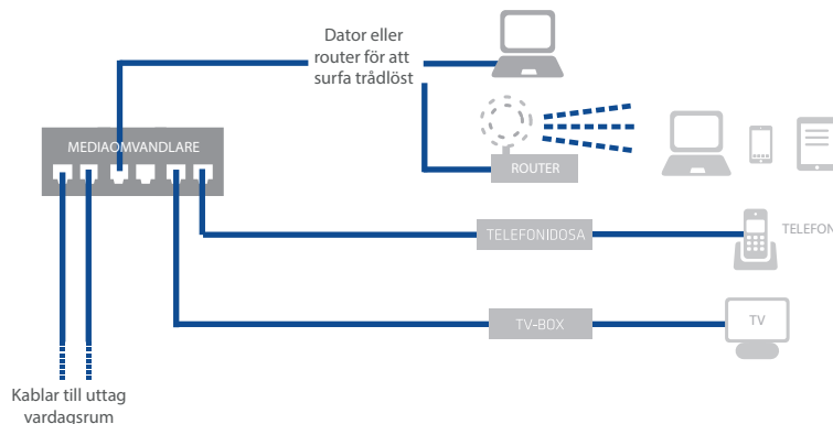
Anslutning från mediaomvandlare i hall
